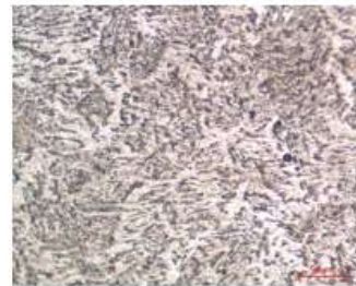
Gambar 4.4.3. foto mikro WM, dengan kuat arus 100 A (normal)
