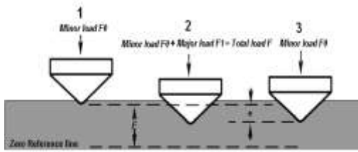
Gambar 2. Skema kondisi indenter
