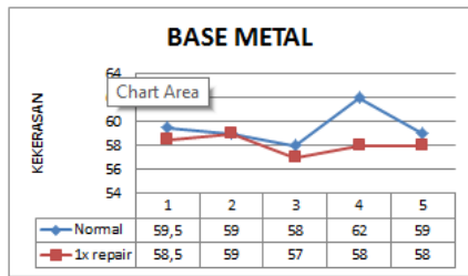
4.3.2 Grafik nilai kekerasan pada base metal dengan kuat arus 100 ampere menunjukkan perubahan kekerasan karena benda uji mengalami deformasi dengan selisih rata-rata 1,4
