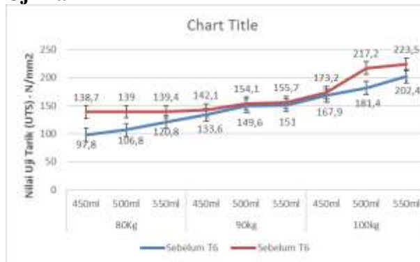
Gambar 6. Grafik hasil uji tarik sebelum T6 dan sesudah T6
