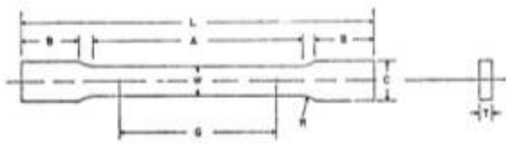
Gambar 2. Spesimen Uji Tarik ASTM E8
