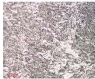
Gambar 4.4.9. foto mikro WM, dengan tegangan 380 V (normal)
