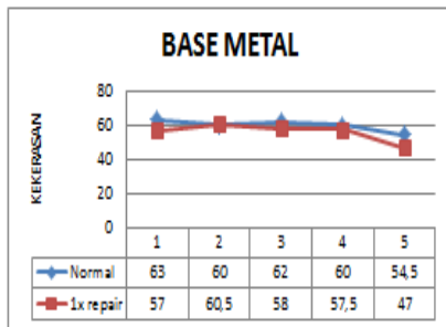
4.3.5 Grafik nilai kekerasan pada base metal dengan tegangan 380 volt menunjukkan perubahan kekerasan karena benda uji mengalami deformasi dengan selisih rata-rata
