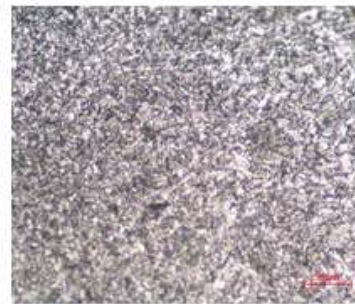
Gambar 4.4.11. foto mikro WM, dengan filler Ø2,6 (normal)
