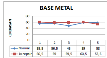
4.3.6 Grafik nilai kekerasan pada base metal dengan filler Ø 2,6 menunjukkan perubahan kekerasan karena benda uji mengalami deformasi dengan selisih rata-rata 3,2
